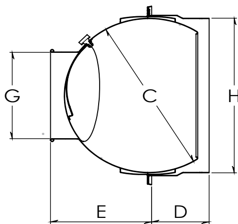
SECCIÓN X-X
